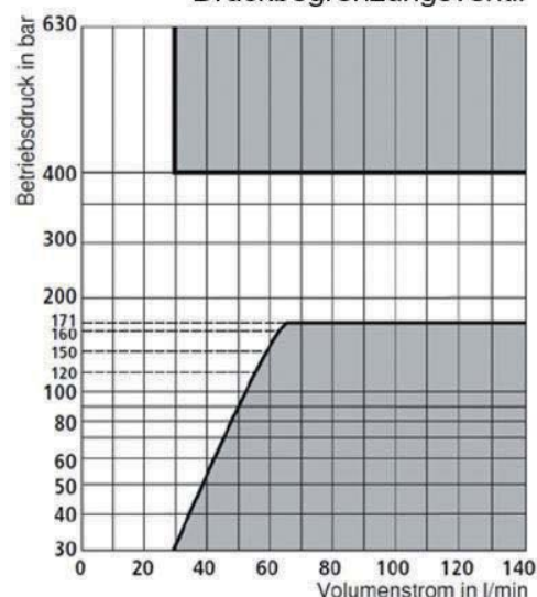
Einsatzgrenzen Druckbegrenzungsventil *
